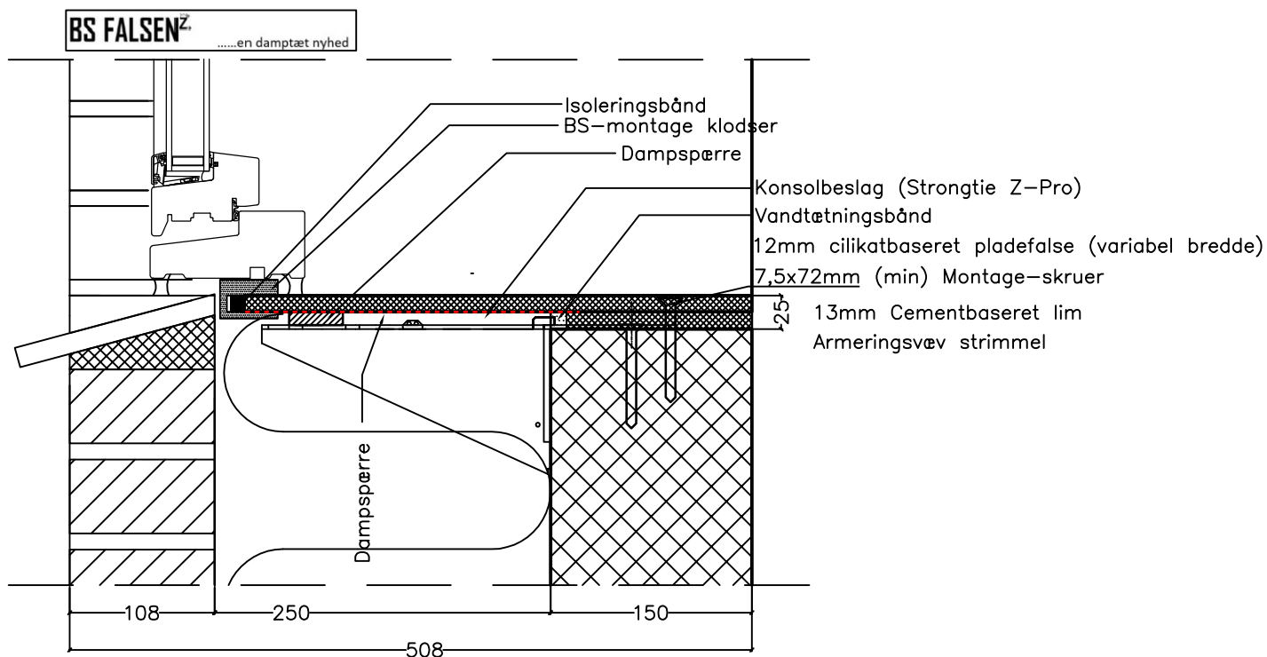
Lodret snit vindue Mur 508 mm
